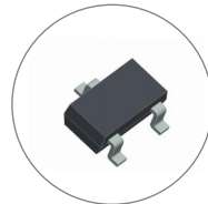
SOT-23-3L(SO) 2.9*1.6*1.1
