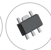
Sot89-5L(SF) 4.5*2.5*1.5
