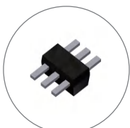
SOT23-6L(SR) 3.0*1.6*1.1
