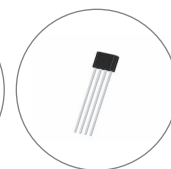
To94-4L(VK) 5.22*3.65*1.56
